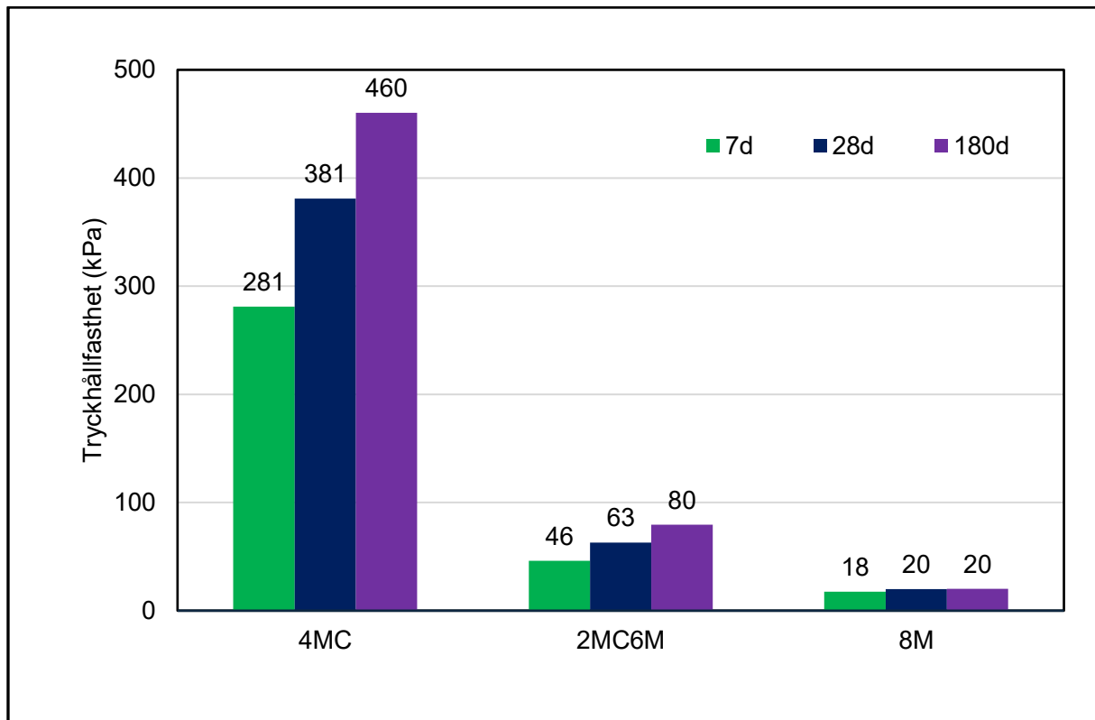
Figur 5.3. Tryckhållfastheten i laboratoriestabiliserad sulfidjord efter olika härdningstid (7, 28 och 180 dagar). Bindemedlen som användes var 4% Multicem (4MC), 2% Multicem + 6% Mesa (2MC6M) och 8% Mesa (8M).
