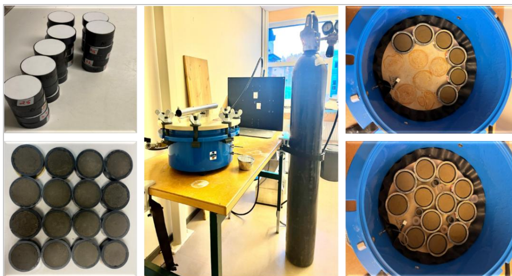
Figur 3.2. Bestämning av jordens vattenhållningsförmåga. Till vänster visas provkroppar före analys. I mitten visas den tryckplatta-kammare som används för att bestämma vattenhållningsförmågan vid olika trycknivåer. Till höger visas provkroppar placerade i kammaren inför mätning. Foto: Abdalla Saafan.
