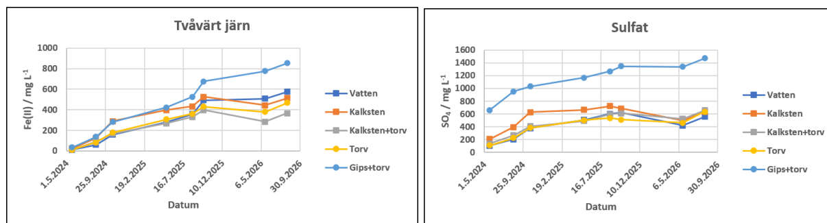
Figur 4.4. Analyserade järn(II)- och sulfathalter i mesokosmrörens markvatten.
