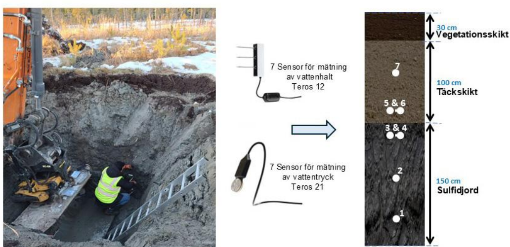
Figur 3.3. Installation av sensorer (fukt och vattenpotential) i sulfidjordcellens täckning vid Umeå deponi och avfallscenter (till vänster). Illustration av markprofilen (till höger). Foto: Ramesh Kumar Thakur.
