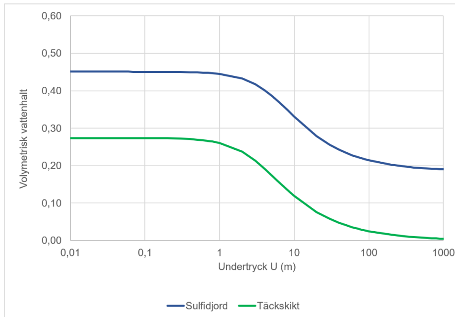
Figur 3.5. Variation av vattenhalten i sulfidjord och täckningsmaterial som en funktion av trycket. Kurvan visar materialens förmåga att hålla vatten. Medan täckningsmaterialet torkar ut håller sulfidjorden kvar vatten vid högt undertryck.
