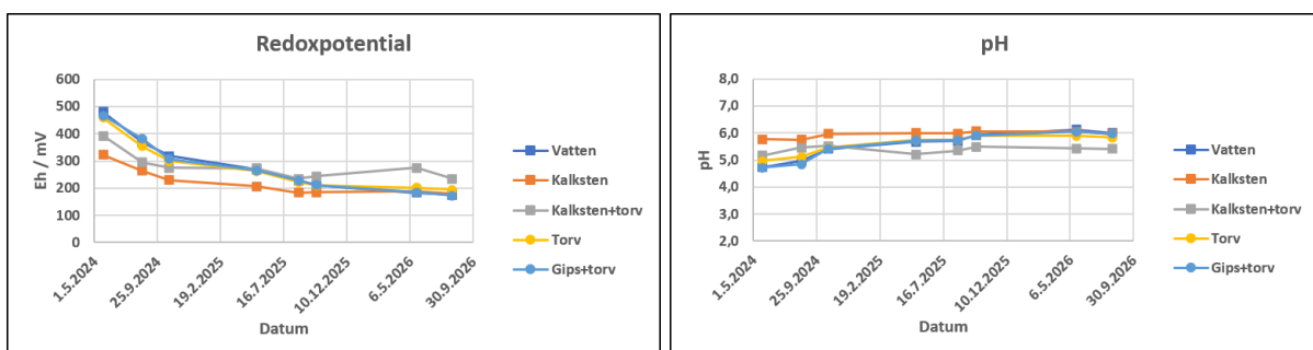
Figur 4.3. Uppmätta redoxpotential och pH-värden från mesokosmrörens markvatten.
