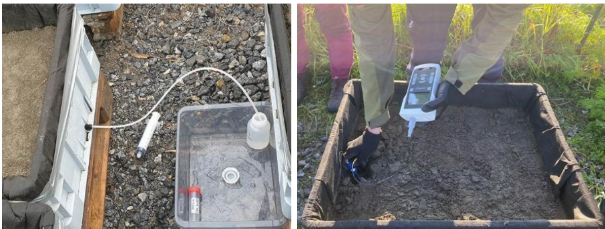
Figur 3.7. Vattenprovtagning från fältförsöket (till vänster) och pH-mätning vid sedimentprovtagningen i fältförsöket (till höger). Foto: Eva Högfors-Rönholm.
